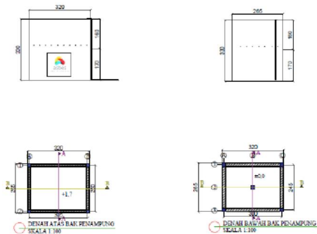
Gambar 5. Denah atas dan bawah bak penampung.
