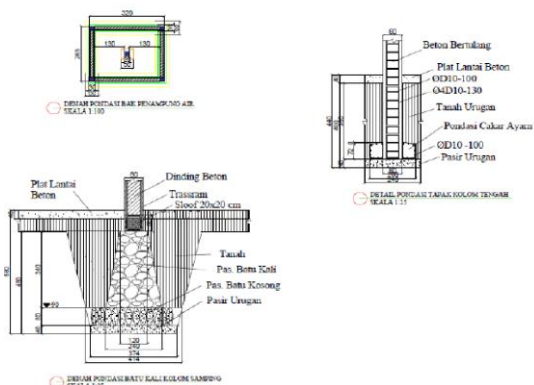
Gambar 6. Tampak samping dan denah pondasi bak penampung.
