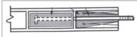
Gambar 7. Pemasangan Mur Baut pada Bambu (Liese, 2003)
