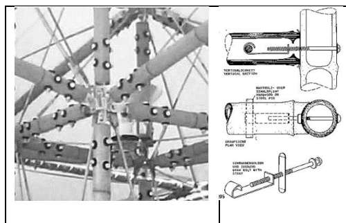
Gambar 6. Sambungan Bambu Menggunakan Baja (Katarzyna, 2013)
