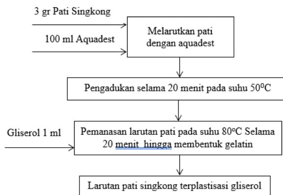
Gambar 1. Diagram alir tahap pembuatan larutan pati terplastisasi gliserol
