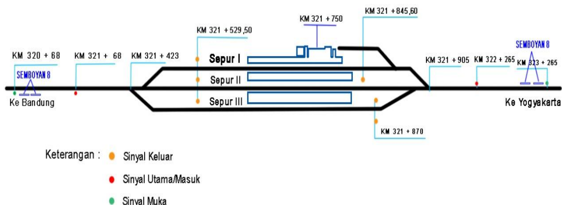
Gambar 1. Denah Emplasemen Stasiun Langen
