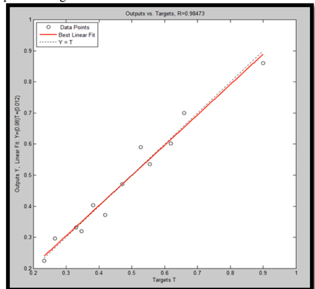
Gambar 6. Grafik Regresi Pengujian Data
