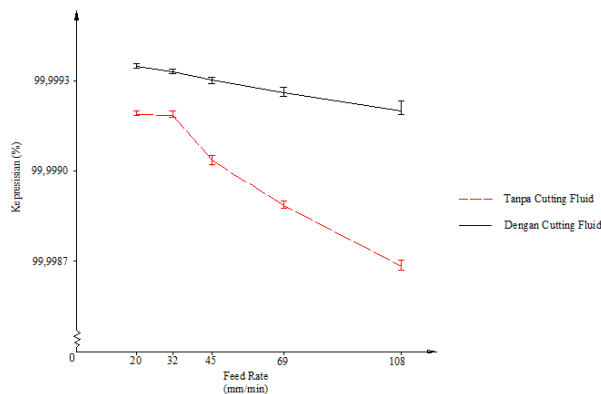
Gambar 4. Grafik Hubungan Feed Rate dengan Kepresisian Data Hasil Pengamatan Dimensi Setengah Lingkaran (A)
