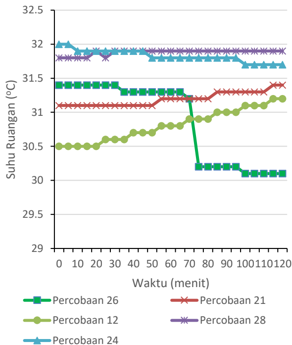
Gambar 8. Grafik Hasil Pengujian Perubahan Suhu Ruang dengan Jarak 2 Meter Terhadap Waktu
