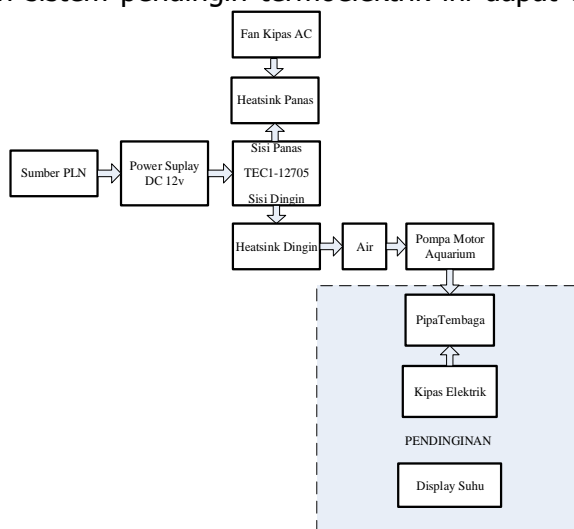
Gambar 2. Diagram Blok Pendingin Ruangan Termoelektrik
