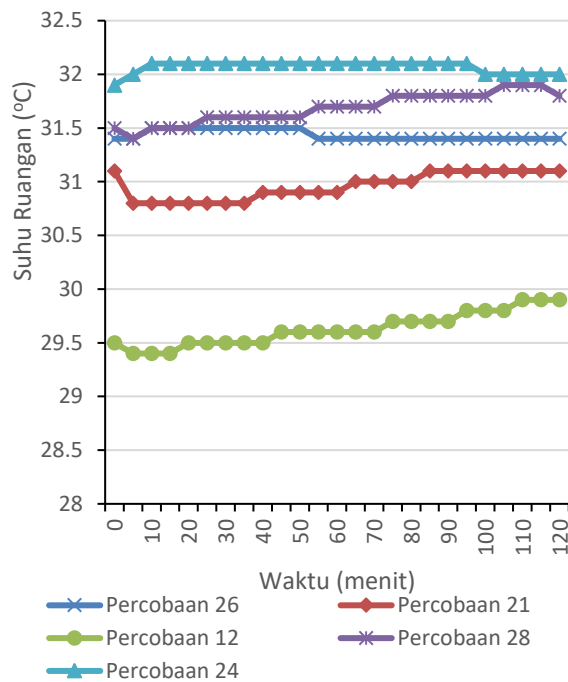
Gambar 7. Grafik Hasil Pengujian Perubahan Suhu Ruang dengan Jarak 1 Meter Terhadap Waktu
