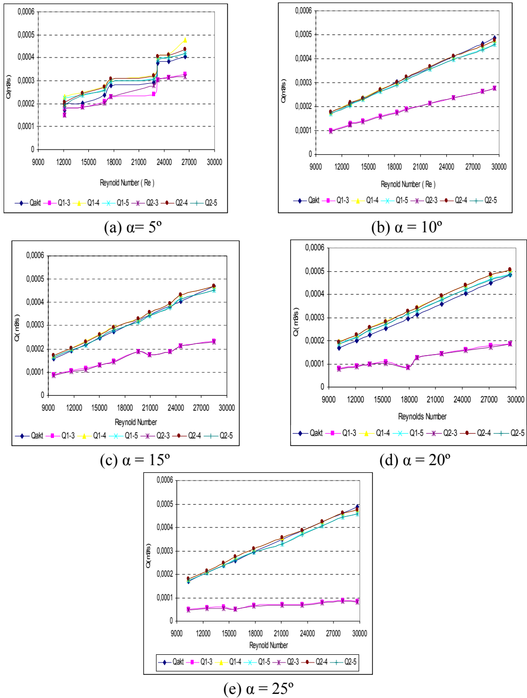
Gambar 7. Grafik perbandingan Q_{akt} terhadap Q_t pada posisi pengukuran \Delta P
