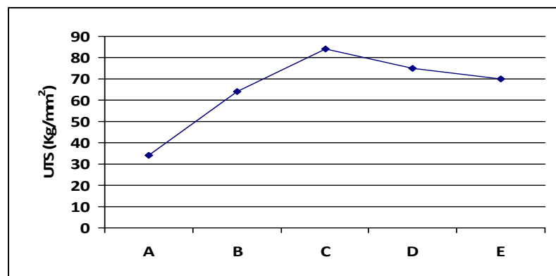
Gambar 1. Grafik Nilai Kekuatan Tarik Tiap – Tiap Sampel 600°C.
