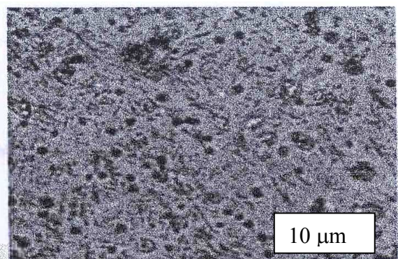
Gambar 4. Foto Struktur Mikro Sampel A 600°C.500X. Gambar 5. Struktur Mikro Sampel D 600°C.500X.
