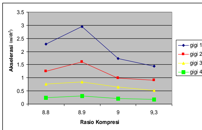
Gambar 2. Variasi rasio kompresi terhadap akselerasi dengan bahan bakar Bensin
