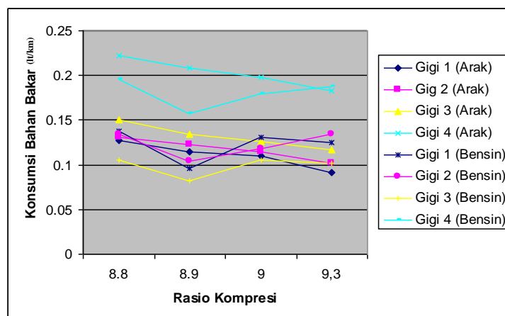
Gambar 6. Perbandingan konsumsi bahan bakar Arak Bali dengan Bensin
