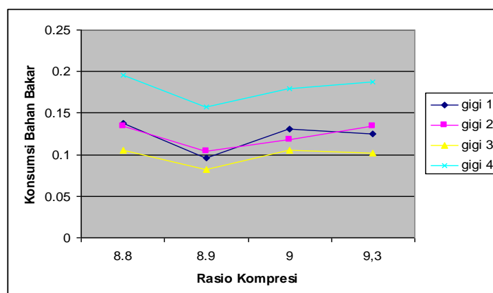
Gambar 4. Variasi rasio kompresi terhadap konsumsi bahan bakar menggunakan bahan bakar bensin
