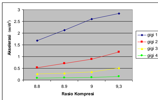
Gambar 1. Variasi rasio kompresi terhadap akselerasi dengan bahan bakar Arak Bali
