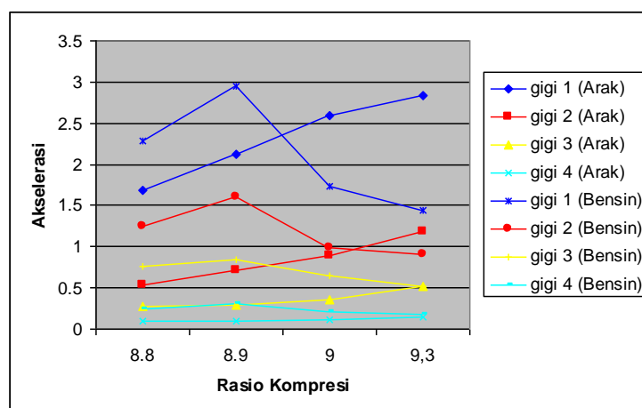
Gambar 5. Perbandingan akselerasi Arak Bali dengan Bensin
