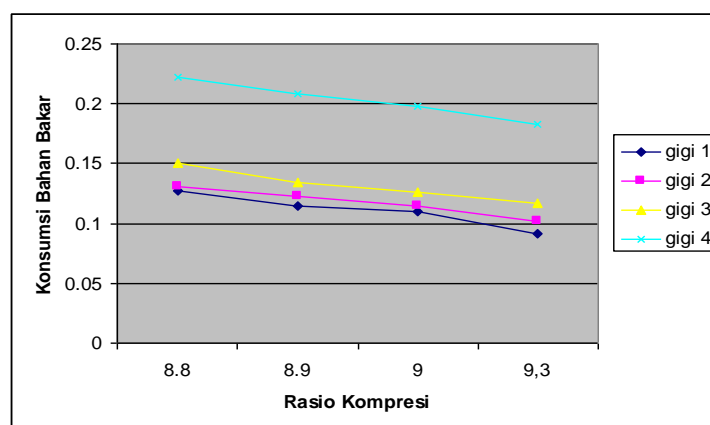
Gambar 3. Variasi rasio kompresi terhadap konsumsi bahan bakar dengan bahan bakar Arak Bali
